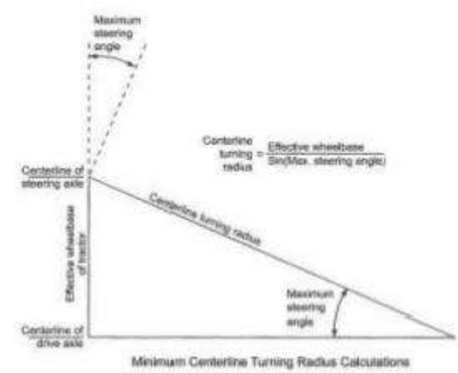
Figura 2-11. Método de cálculo para determinar el radio de inflexión en línea central Camiones tractor-Semirremolque
