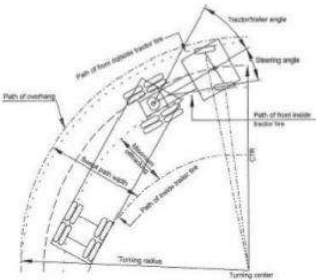
Figura 2-10. Características de giro de una combinación típica Camión Tractor-Semirremolque
